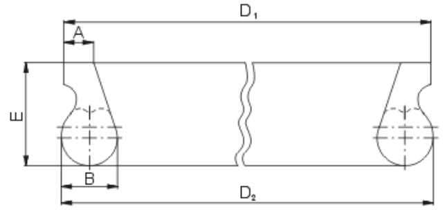
■ DN 100~600 mm
