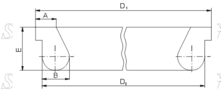
■ DN 700~2000 mm
